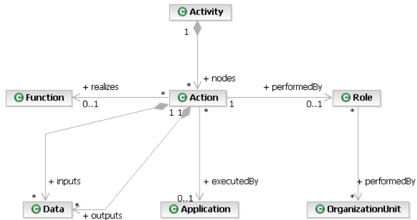
Abbildung 9: Domänen-spezifisches Modell: Funktionen, Rollen, Anwendungen und Daten
