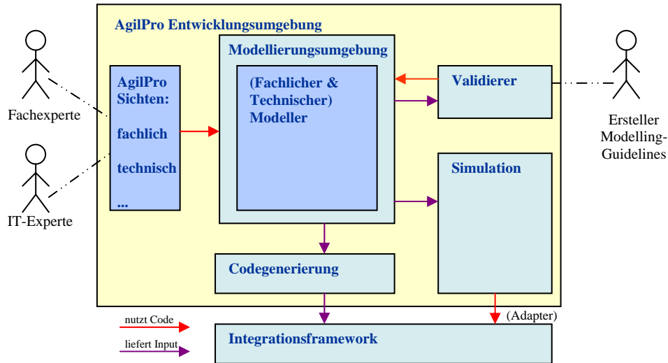
Abbildung 5: Aufbau der AgilPro-Entwicklungsumgebung
