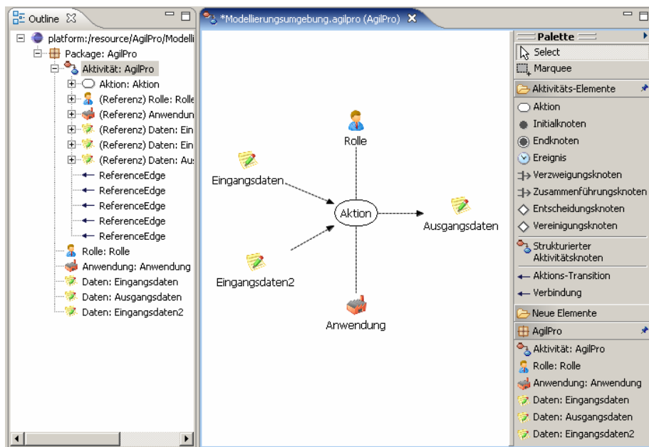
Abbildung 6: AgilPro Modellierungsumgebung
