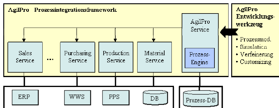
Abbildung 4: Übersicht über den Aufbau von AgilPro
