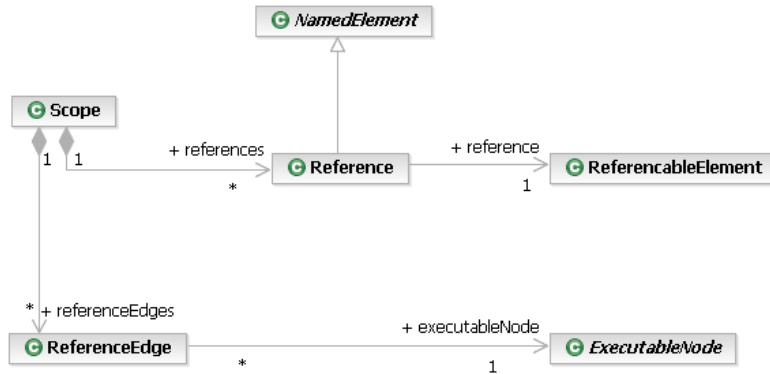
Abbildung 8: Domänen-spezifisches Modell: Referenzen
