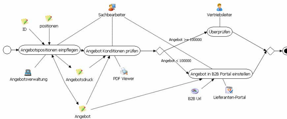
Abbildung 1: Beispiel eines Prozesses in AgilPro
