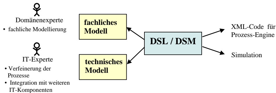
Abbildung 3: Modellierung verschiedener Sichten
