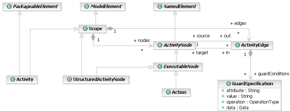
Abbildung 7: Domänen-spezifisches Modell: Prozesse
